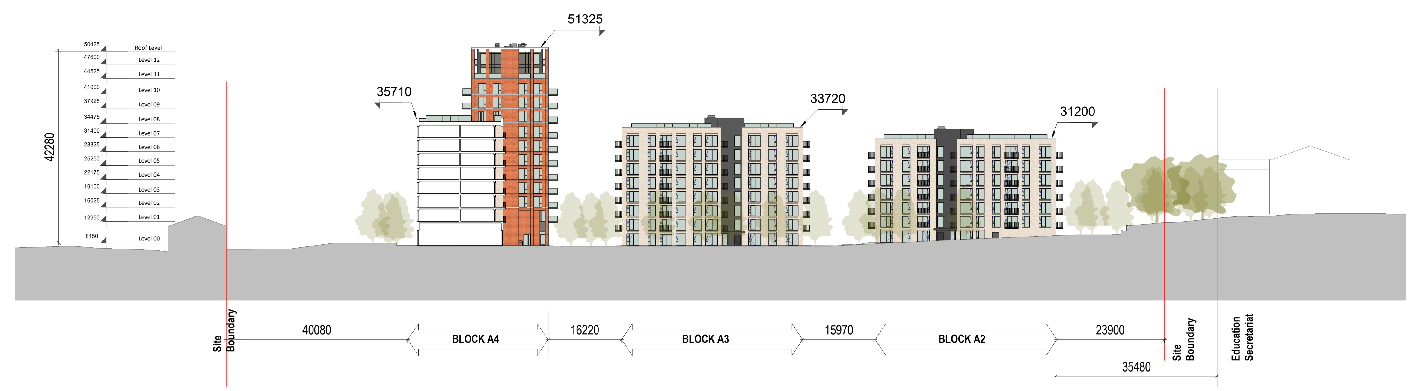
④ Site Section 1 1:500
